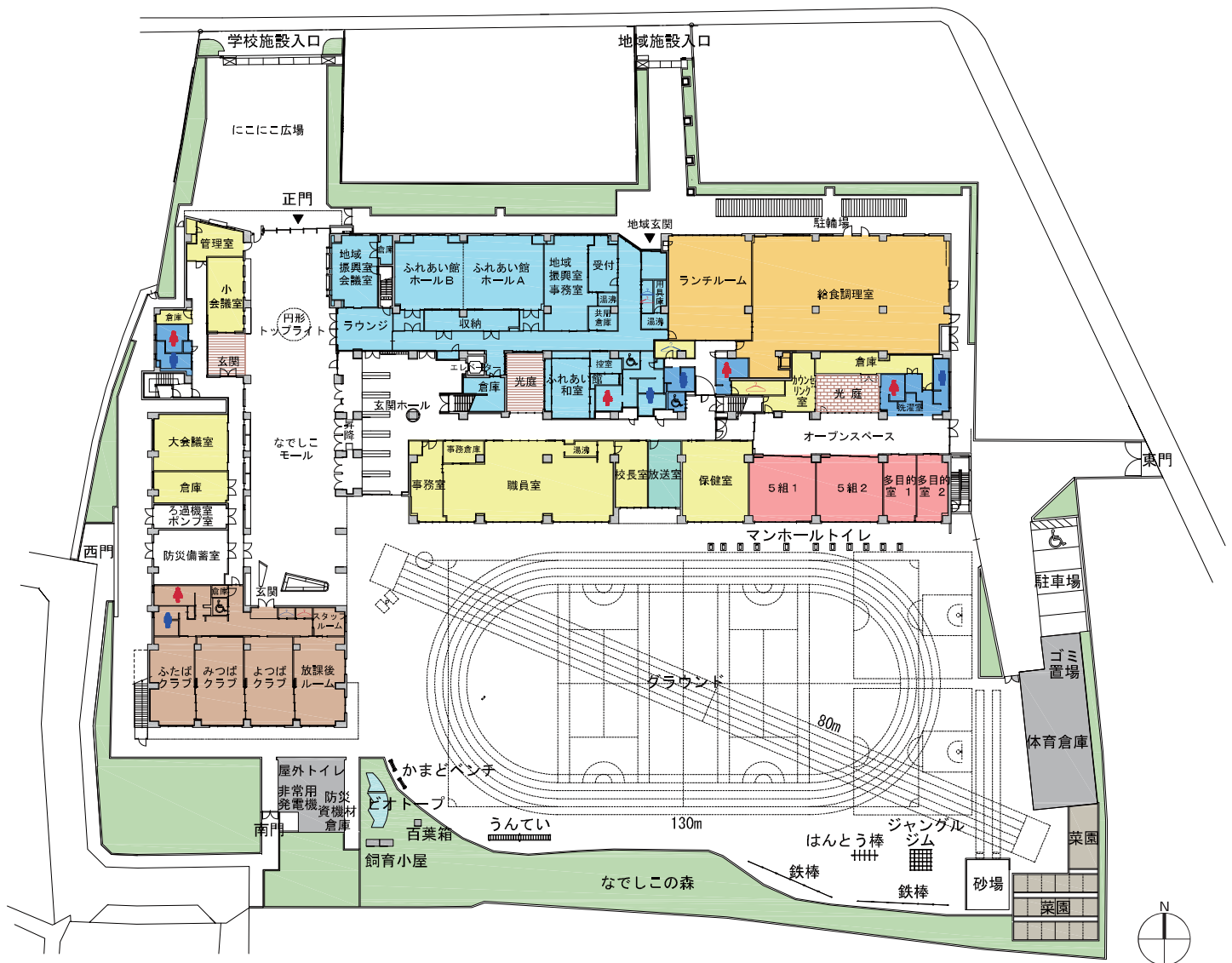
1階平面図
