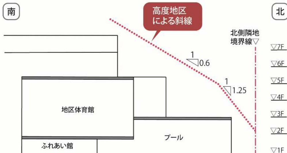
C断面
