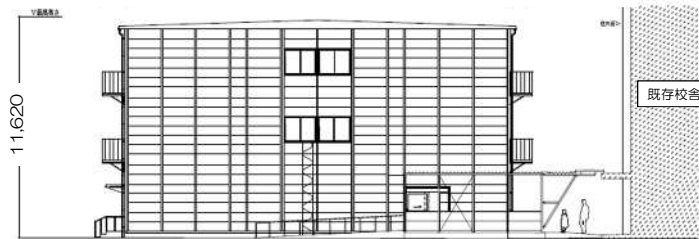
東側立面図
