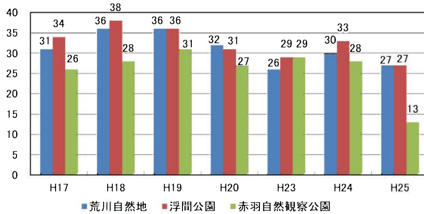
図 23 区内で確認された野鳥の種類数の推移
