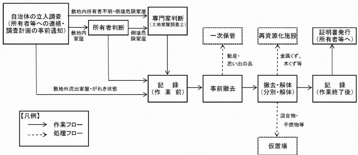
図 2-8 公費解体作業フロー及びがれき処理フロー
